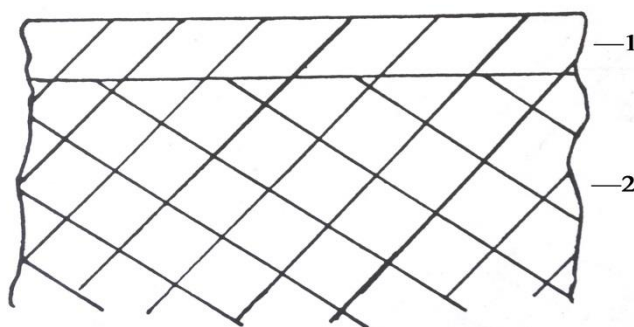
Рис. 3 Разрез поверхности мохового болота, где: 1-сухой слой, 2-влажный.
